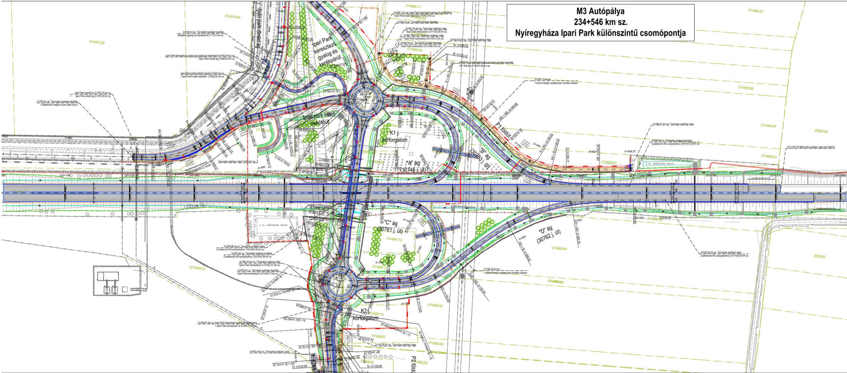
Nyíregyháza Ipari Park bővítése – M3 autópálya új különbsztű csomópont – Általános helyszínrajz - részlet Tervező: CÍVIS KOMPLEX MÉRNÖK Kft. (4034 Debrecen, Nagybánya u. 17.)
